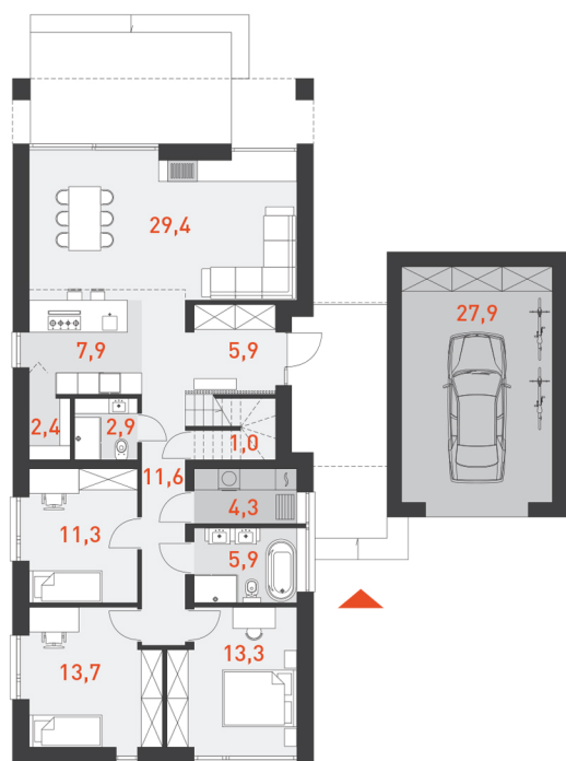
RZUT PARTERU 105,3 m 2
